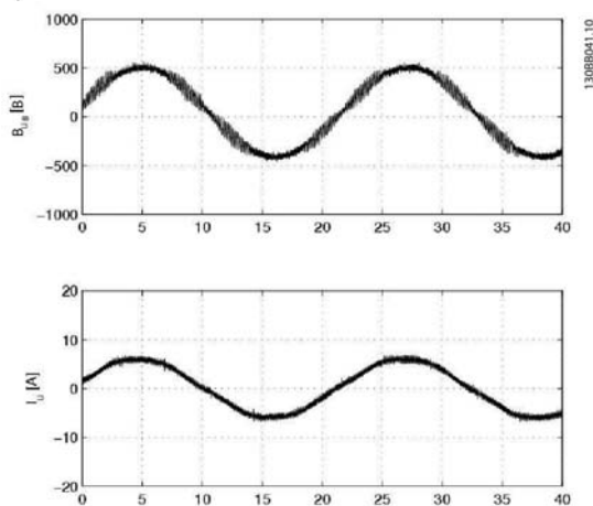
Рис. 3.15 Напряжение и ток с синусоидальным фильтром
