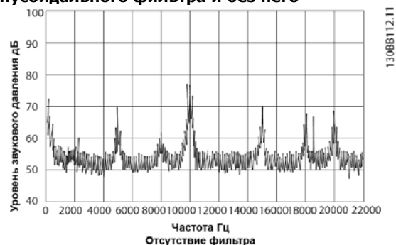
Отсутствие фильтра
