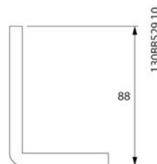
Рис. 5.16 Комплект L-образных клемм 130B3138
