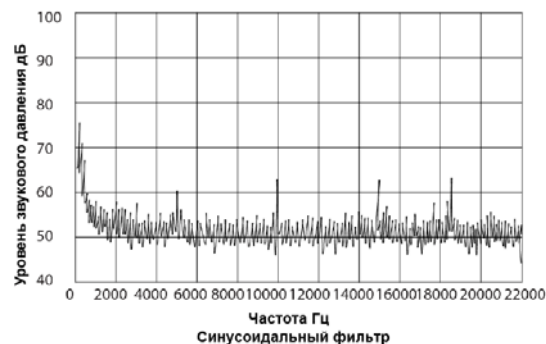
Синусоидальный фильтр
