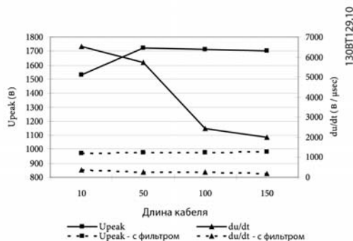
Рис. 3.13 690 В – С фильтром dU/dt и без него
